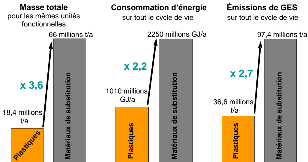
Figure 1 : Effet du remplacement de certains emballages plastiques sur les masses, la consommation énergétique et les émissions de GES
